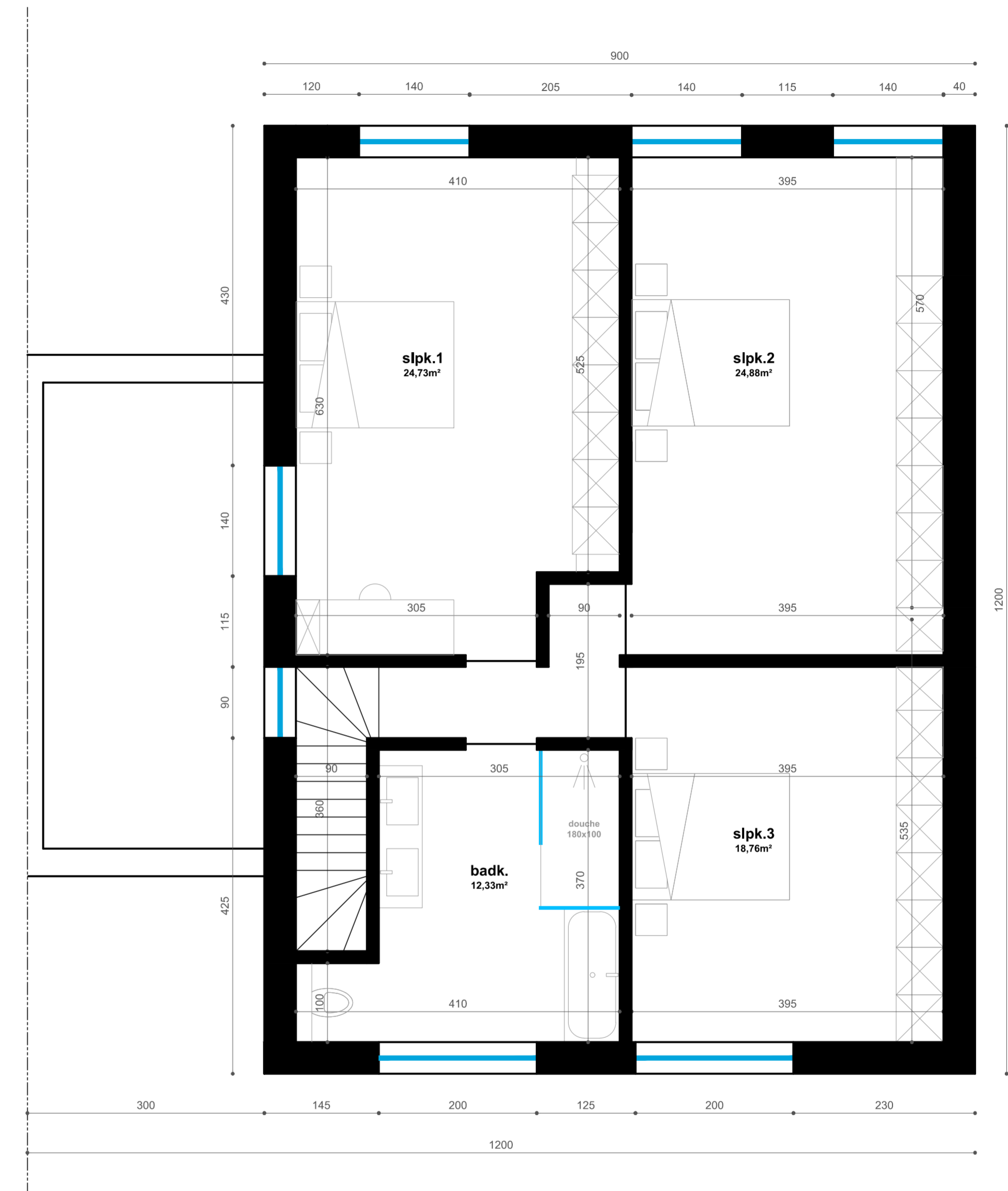
VERDIEPING nieuwe toestand schaal 1/50
