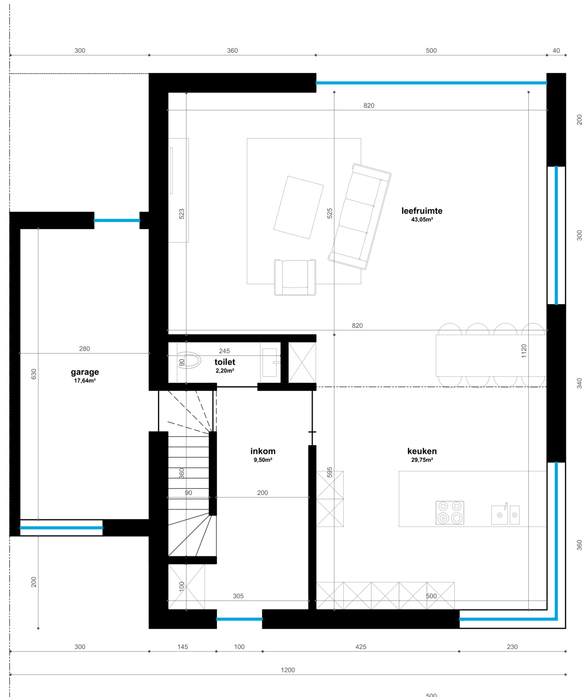
GELIJKVLOERS nieuwe toestand schaal 1/50
