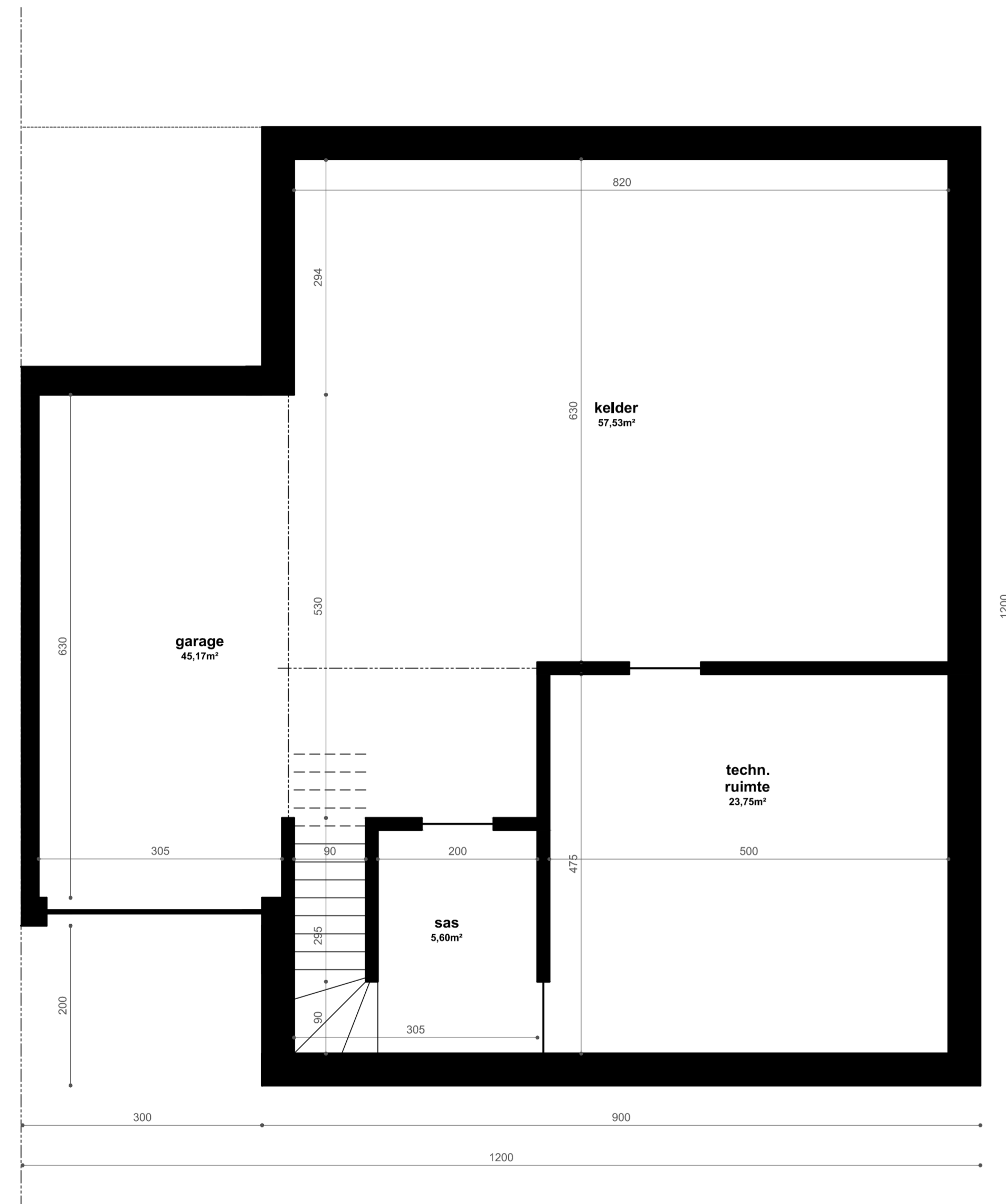
KELDER nieuwe toestand schaal 1/50
